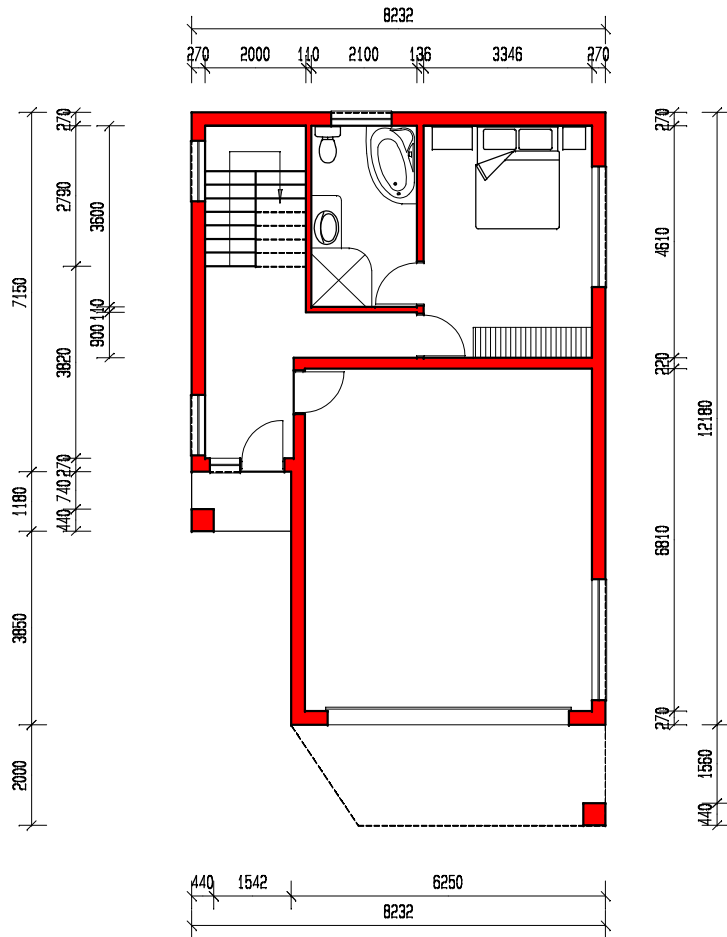
GRONDVLOER VERDIEPING SKAAL 1:100
