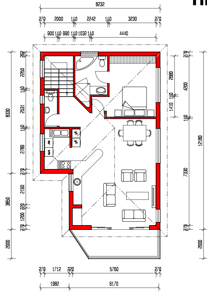
EERSTE VERDIEPING SKAAL 1:100
